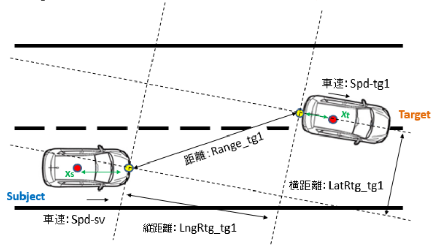
&lt;Target車両の進行方向の座標系&gt;
