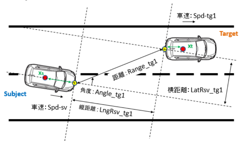
&lt;Subject車両の進行方向の座標系&gt;
